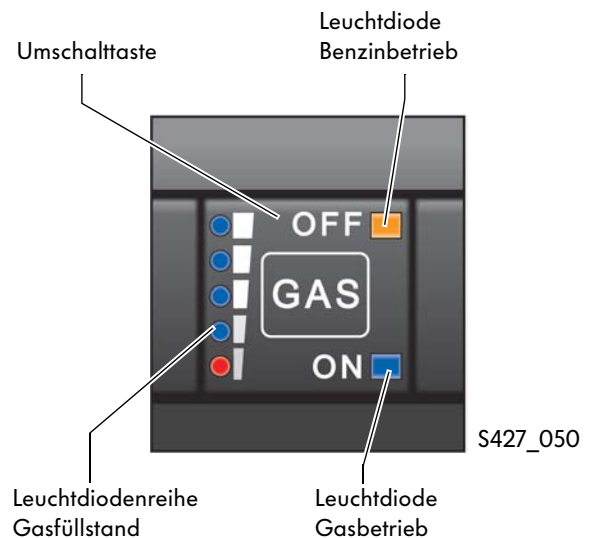
Umschalttaste mit Gasvorratsanzeige G706 und Schalter für Kraftstoffauswahl E395
